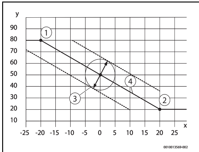
Obr. 4 Ekvitermní křivka
