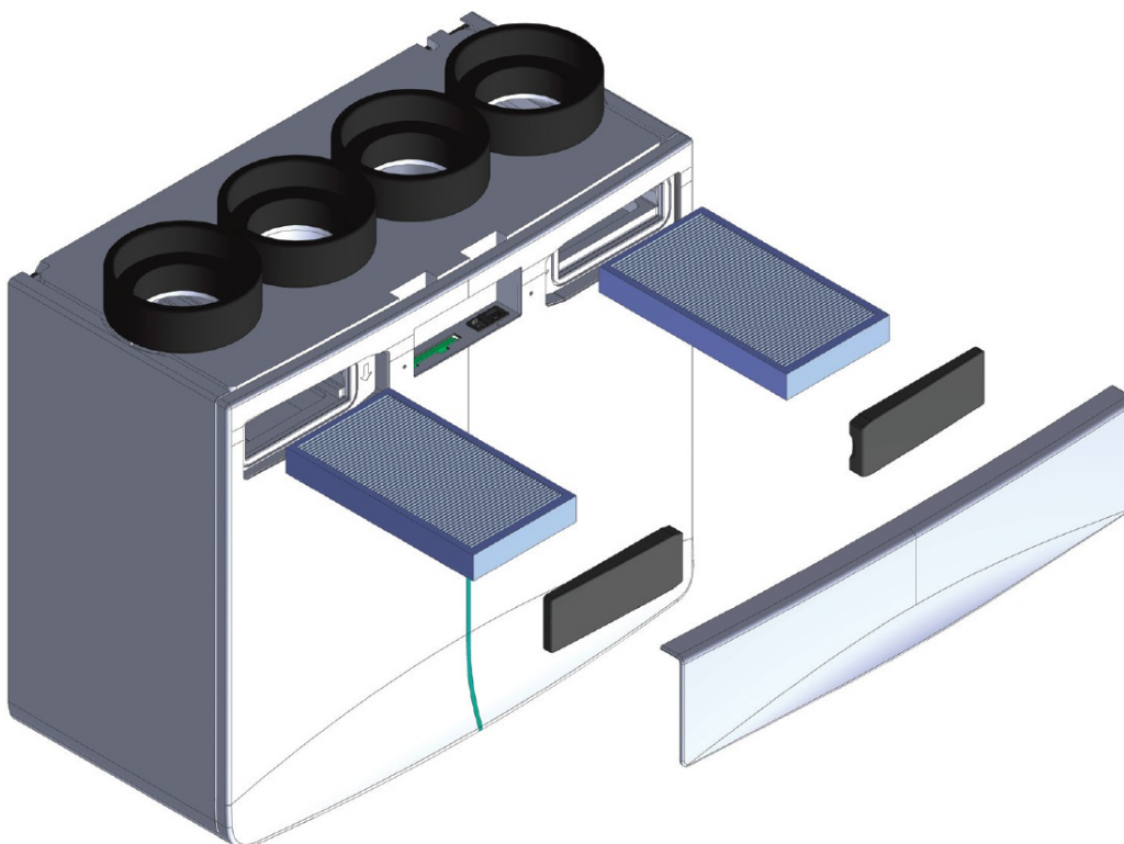
Obrázek 5 – Výměna filtrů
