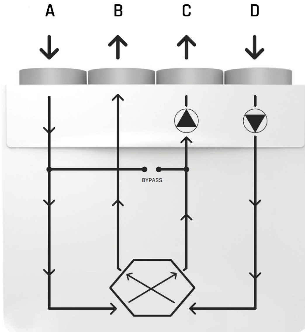
Obrázek 2 – Princip rekuperace
