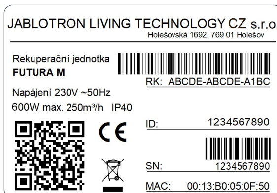
Obrázek 1 – Identifikační štítek
