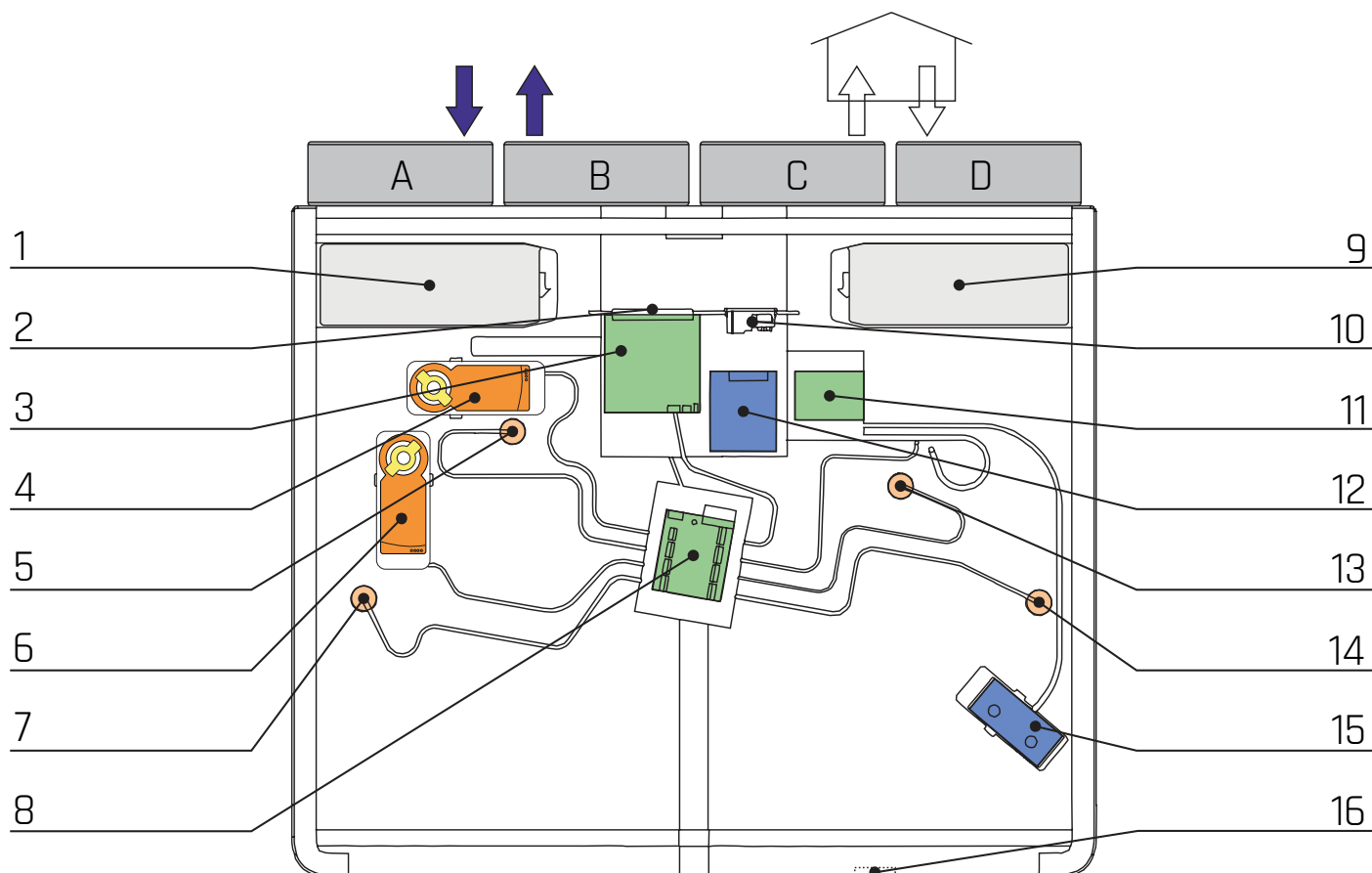
Obrázek 3 - Konstrukce zařízení
